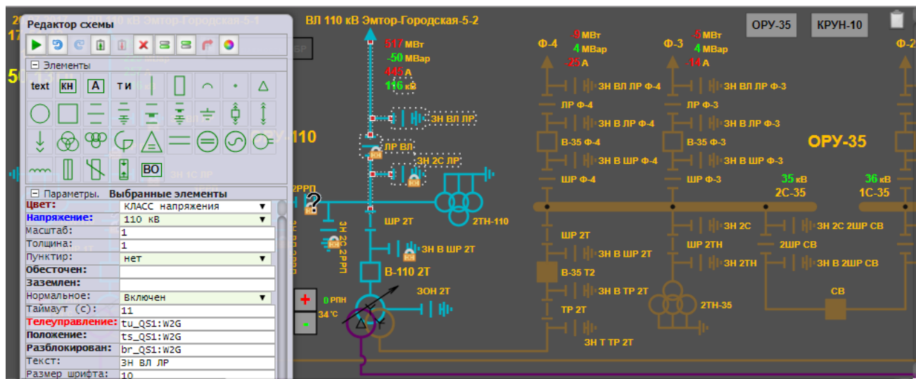
Рисунок 2 Редактор схемы
